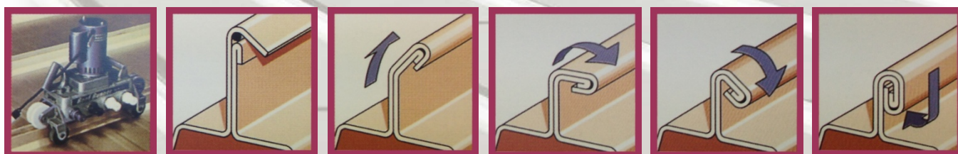
Proceso de engatillado del MR-24
